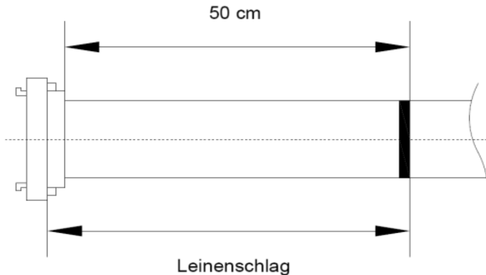
Abb. 10: Anbringung der Markierung auf dem Saugschlauch und schematische Darstellung des Bereiches für den Leinenschlag
