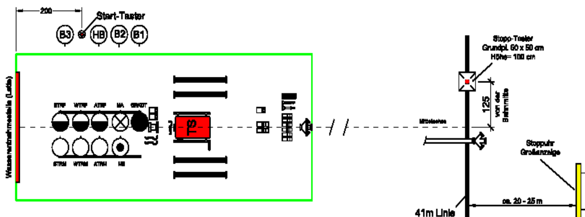
Abb. 27 Aufbau der elektronischen Zeitnehmung
